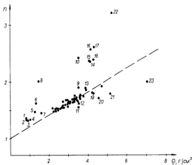
Рис. 11. Зависимость между коэффициентом преломления n и плотностью \rho некоторых жидких и твердых веществ, минералов (составлено по данным [55, 57]). 1 — лед, 2 — ацетон, 3 — спирт, 4 — вода, 5 — глицерин, 6 — сероуглерод, 7 — четыреххлористый углерод, 8 — сера, 9 — титанит, 10 — алмаз, 11 — гротит, 12 — топаз.
