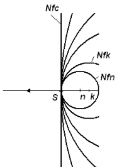
Рис. 22. Образование фронта электромагнитной волны от источника, движущегося со скоростью V равной скорости C .
