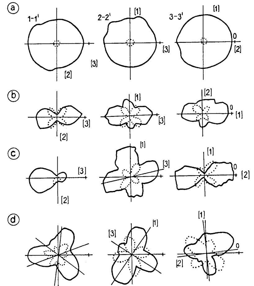
Рис. 2. Акустополяриграммы кубических образцов силикатного стекла (а), дерева (б), монокристалла микролина (с), синтетического кварца (д) в трех взаимноперпендикулярных направлениях 1-1', 2-2', 3-3'. Сплошная линия - векторы параллельны, пунктир - векторы скрещены.
